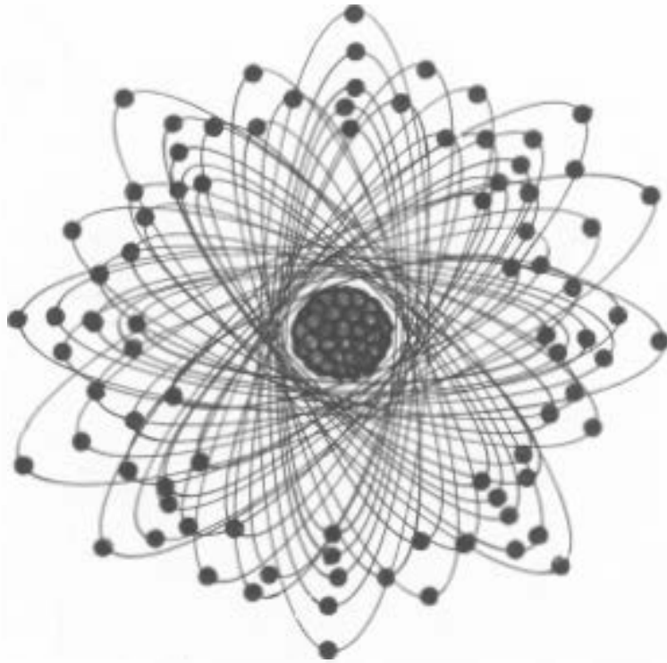
Uranium atom
